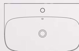
Art. 5508 - 70 x 45 x h15 cm MOON 70R H15
